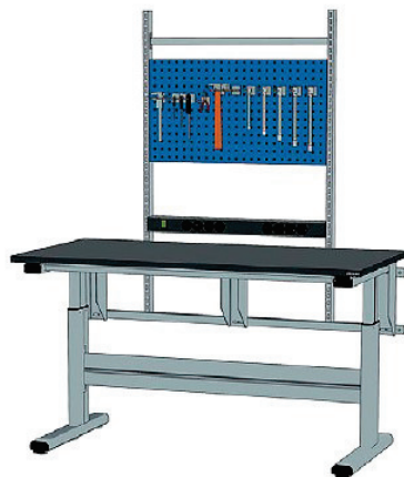
Perf. Stolpe højde 1446 mm. c/c 900
